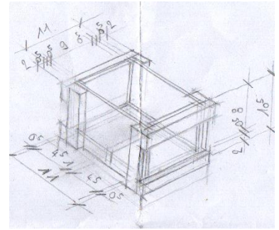
Abb. 43 Musterkonzeption Silikonersatz Skizze 13.02.2020
