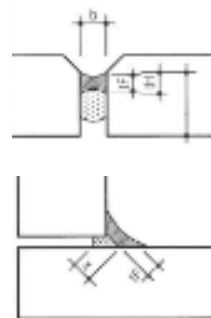
Abb. 42 Stoss-, und Winkelfuge Schulungsunterlagen Konstruktionslehre Bauberufe
